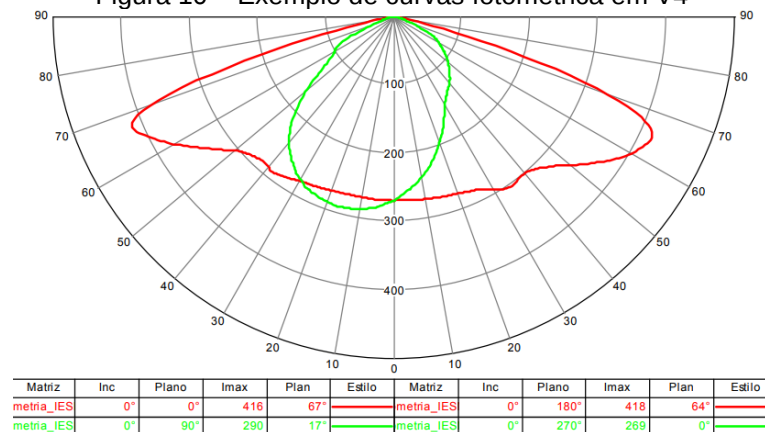
Figura 10 – Exemplo de curvas fotométrica em V4
