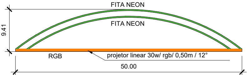
VISTA PONTE ESC.: 1/500 FITA NEON - 240m projektor linear rgb 200unidades
