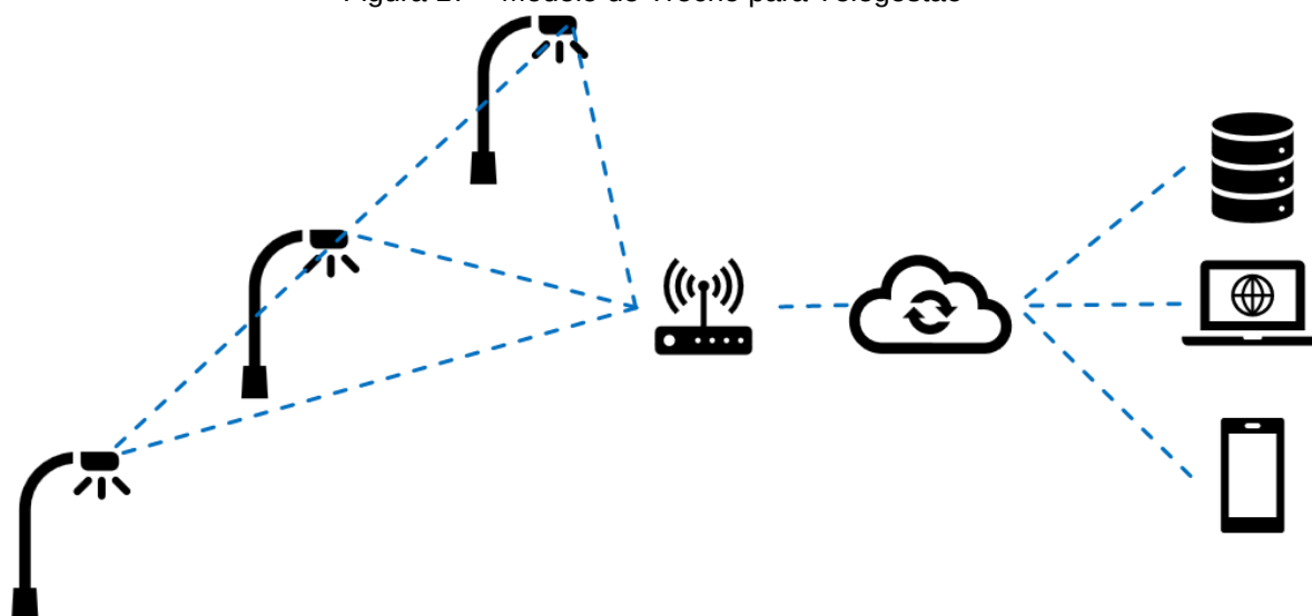
Figura 17 – Modelo de Trecho para Telegestão
