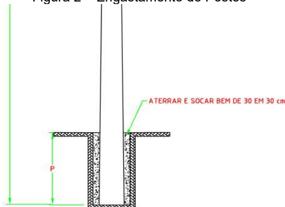
Figura 2 – Engastamento de Postes
